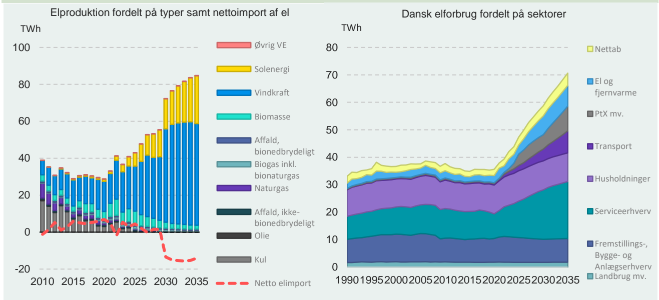
FIGUR 6. FORUDSAT VÆKST I ELFORBRUG OG ELPRODUKTION
