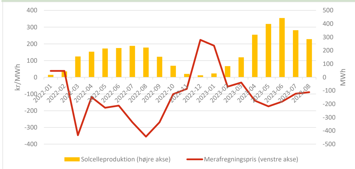
FIGUR 10. SOLCELLEPRODUKTION OG FORSKEL MELLEMLIG GENNEMSNITLIG STRØMSPRIS OG AFREGNINGSPRIS FOR SOL
