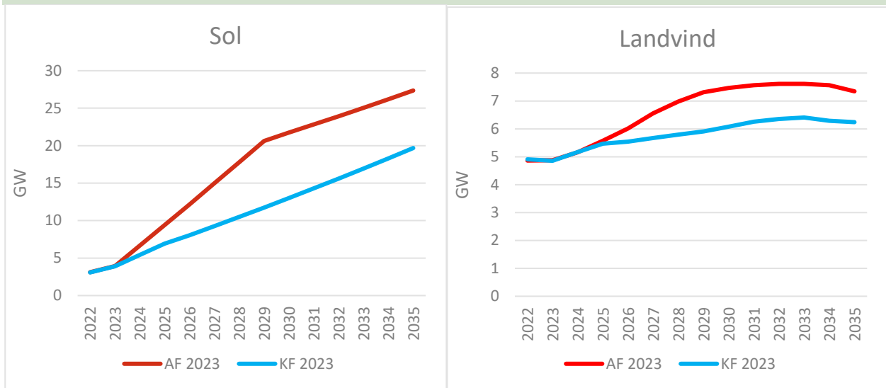
FIGUR 5. FORUDSAT VÆKST I SOL- OG LANDVIND-KAPACITET
